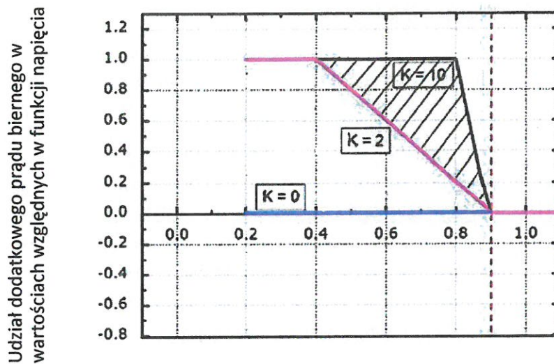
Wartość napięcia na zaciskach podstawowej instalacji wytwórczej
